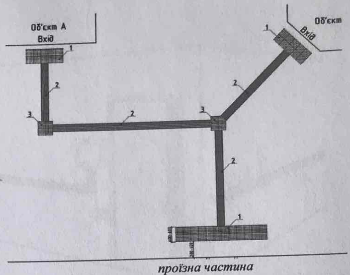
Рис. 7. Приклад улаштування тактильних смуг (ТС): 1 - попереджувальна ТС; 2 - направляюча ТС; 3 - інформаційна ТС, яка вказує місце повороту (розходження) направляючої ТС
