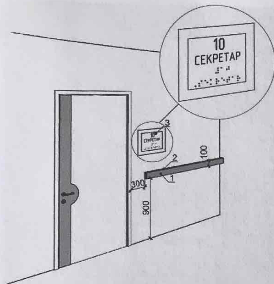
Рис. 8. Приклад розміщення тактильних інформаційних покажчиків приміщень: 1 - інформаційна направляюча; 2 - тактильна інформаційна позначка; 3 - інформаційна тактильна табличка, що дублює текстову інформацію у тактильному вигляді плоско-друкованого тексту та шрифтом Брайля
