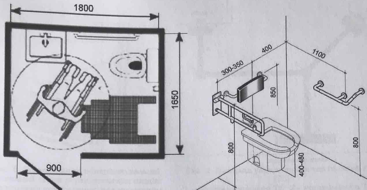
Рис. 5. Обладнання універсальної kabіни. План, загальний вигляд
