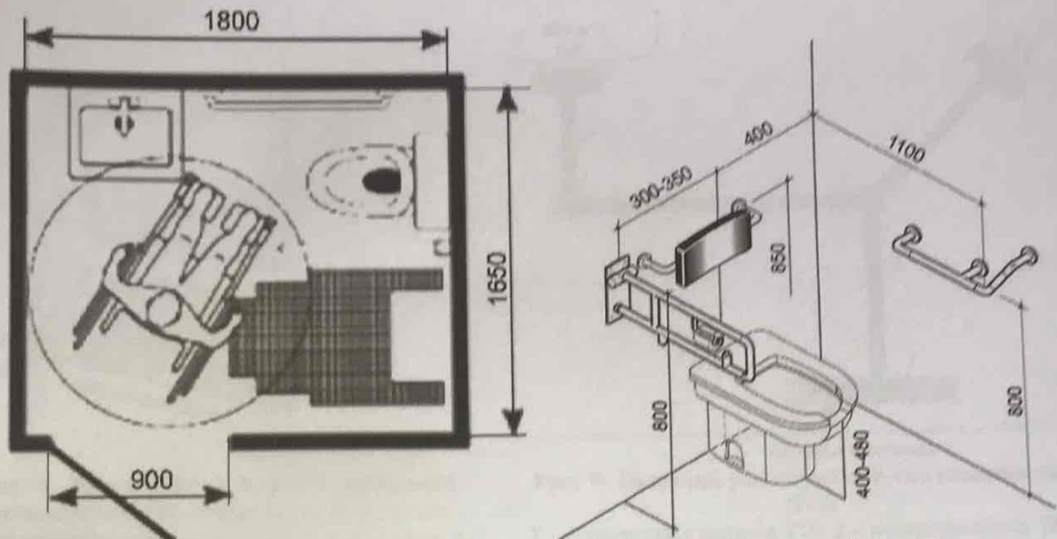
Рис. 7. Обладнання універсальної kabіни. План, загальний вигляд
