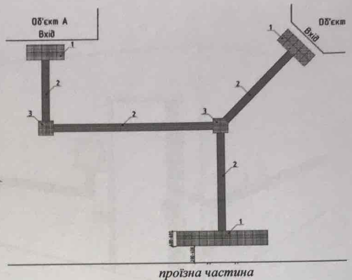
Рис. 9. Приклад улаштування тактильних смуг (ТС): 1 - попереджувальна ТС; 2 - направляюча ТС; 3 - інформаційна ТС, яка вказує місце повороту (розходження) направляючої ТС
