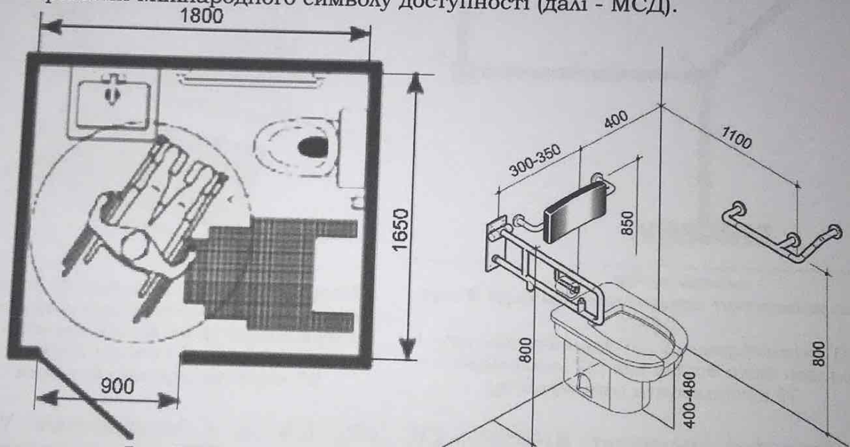
Рис. 7. Обладнання універсальної кабіни. План, загальний вигляд
